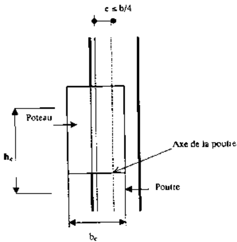
Figure 7.3 : Excentricité des axes poteau-poutre
