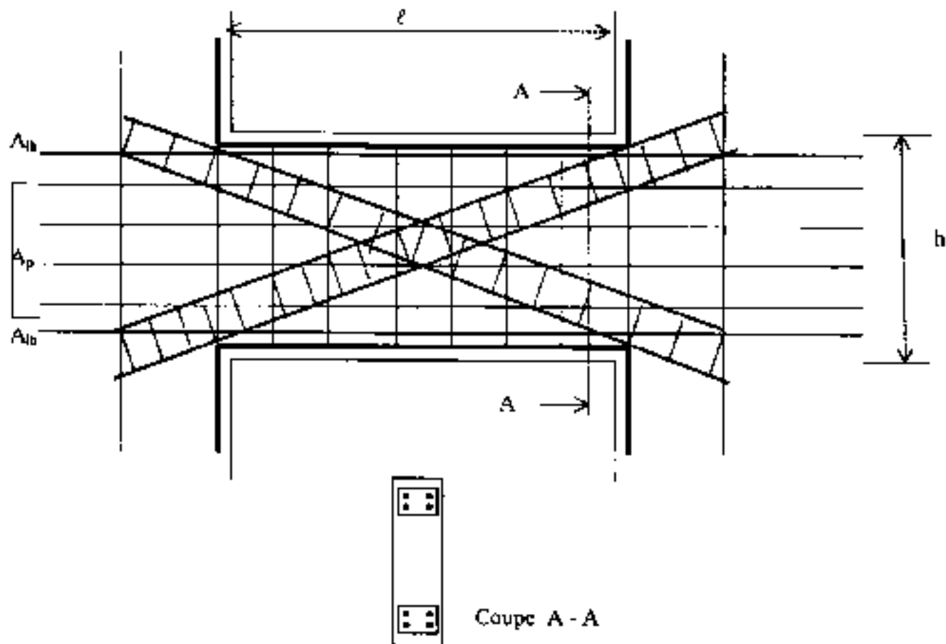
Figure 7.9 : Ferrailage du Linteau
