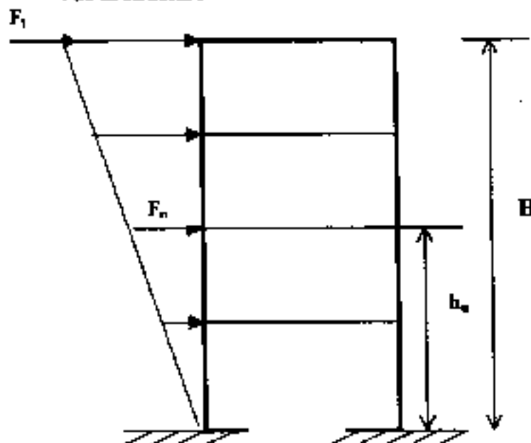
Figure 6.1 : Répartition verticale des forces sismiques
